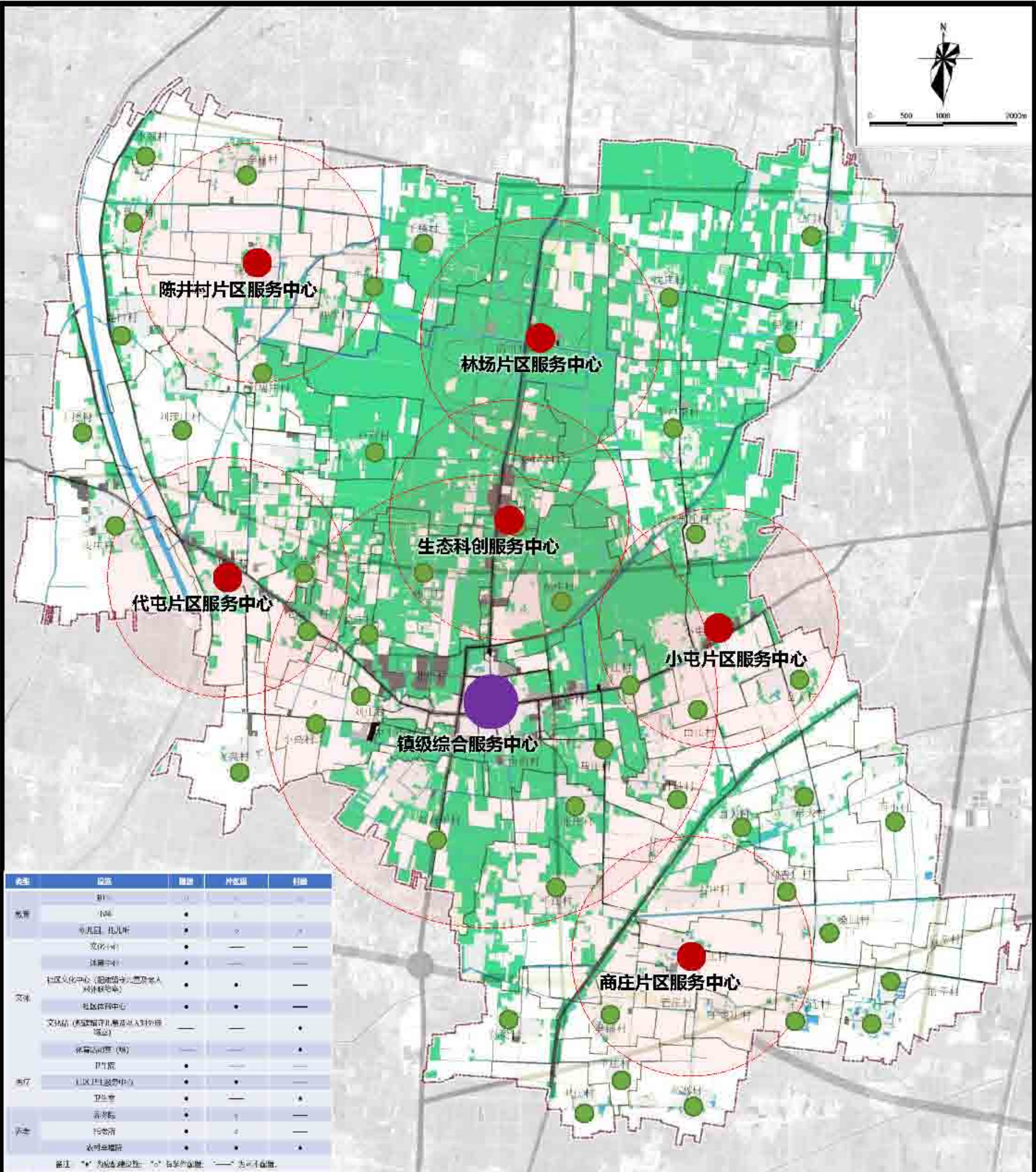
镇域服务设施提升规划图
