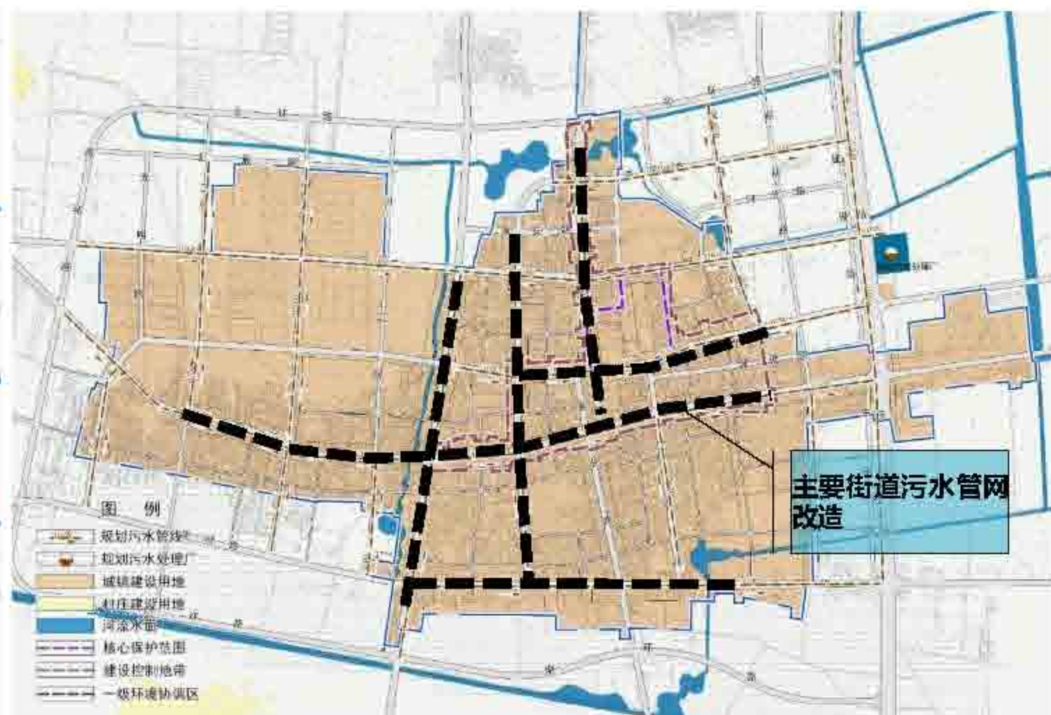
镇区污水工程规划图
